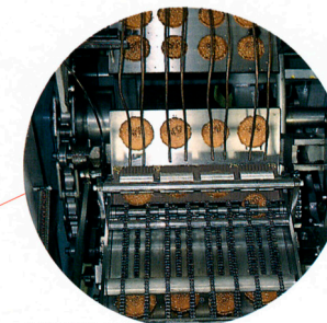
▲自動製品取だし装置
